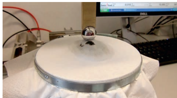
Reisst das Tuch schnell? Dazu wurden die Taschentücher in ein Druckprüfgerät gespannt
